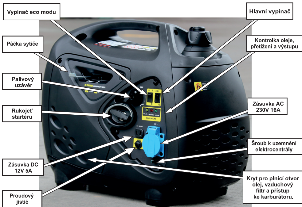
Obr. jednofázové elektrocentrály PH-PROGRESS COMPACT 1000
